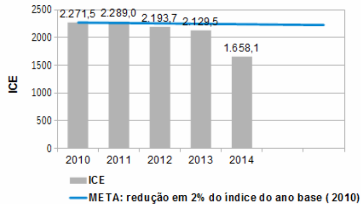
INDICADOR 5 - ÍNDICE DE CONSUMO DE ENERGIA ELÉTRICA (ICE)
