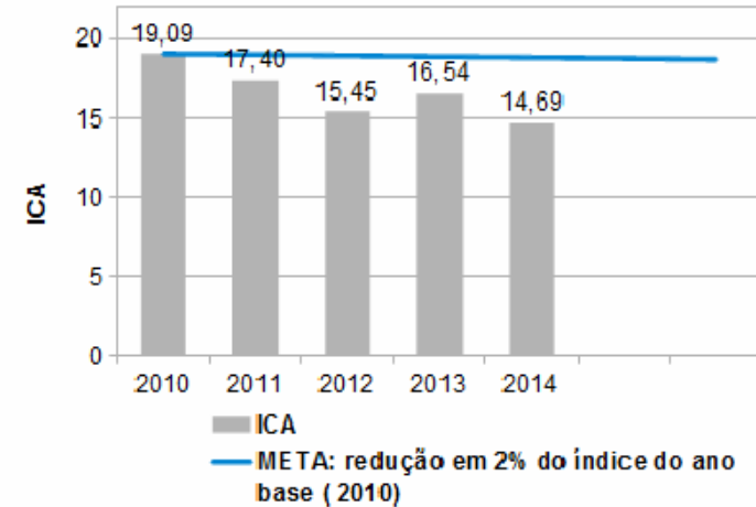
INDICADOR 6 - ÍNDICE DE CONSUMO DE ÁGUA (ICA)
