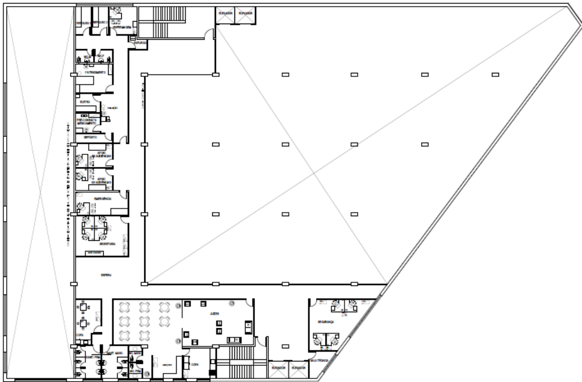
PLANTA DO 1º PAVIMENTO
